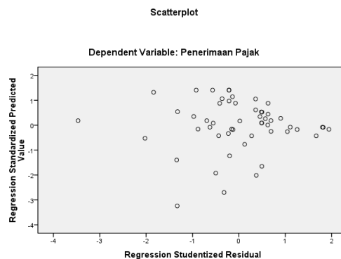
Gambar 2. Grafik scatterplot hasil uji heteroskedasitas
