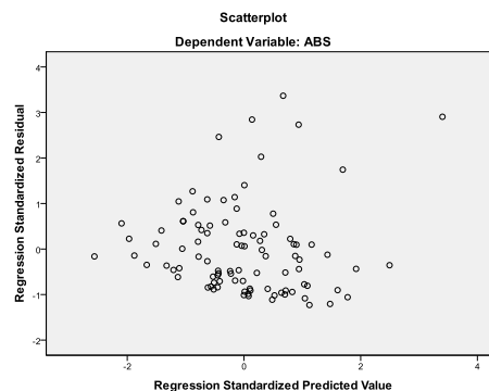
Gambar 1. Uji Heterokedastisitas Sumber : Hasil Pengolahan Data SPSS
