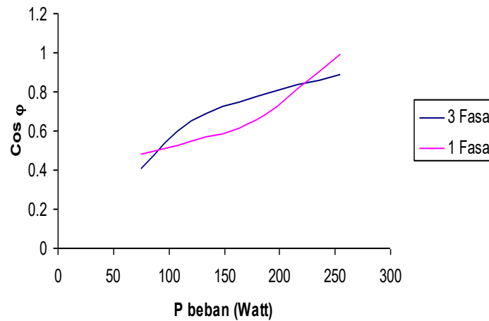
Gambar 5 Karakteristik hubungan \cos \phi terhadap beban motor
