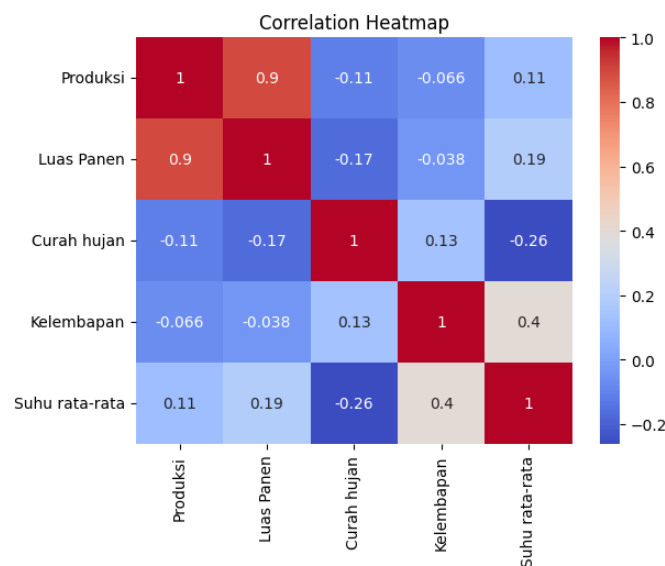
Gambar 5 Matriks Korelasi
